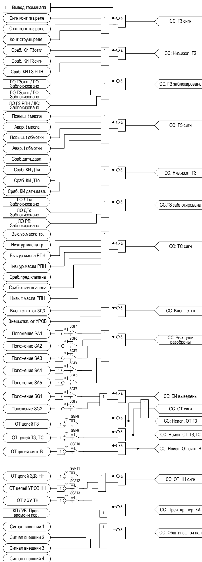
Рисунок 2.34 – Функциональная схема сборки сигналов
